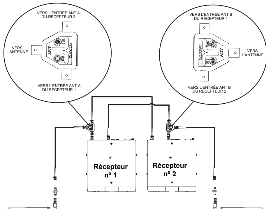
RACCORDEMENT DES COUPLEURS D'ANTENNES UA221 FIGURE 1
